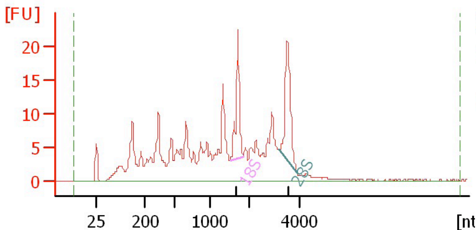
降解的RNA在低分子质量处显示为曳尾 (smear)
