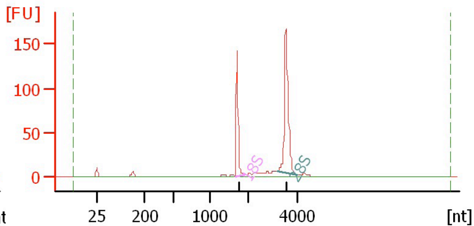
完整的总RNA显示陡峭的28S和18S rRNA峰
